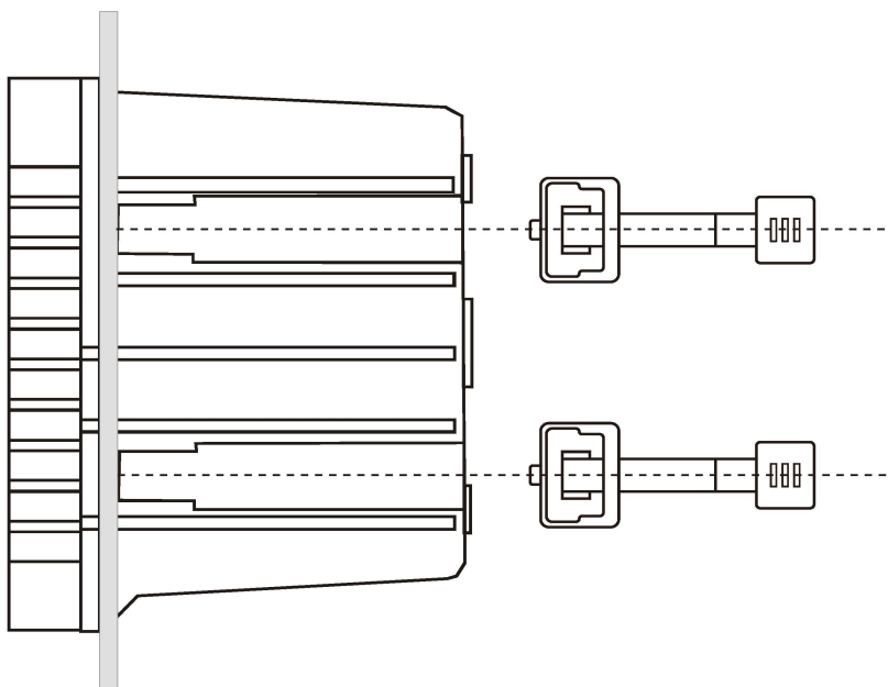
144 系列支架安裝圖
